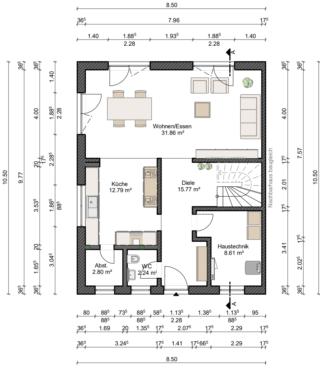
ERDGESCHOSS M 1:100
